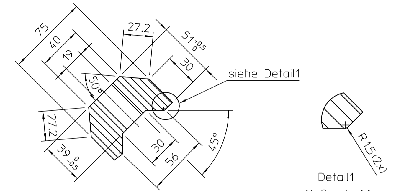
Schnitt D-D
