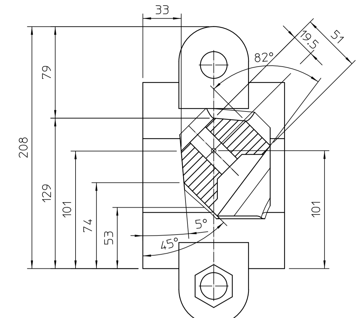
Schnitt C-C
