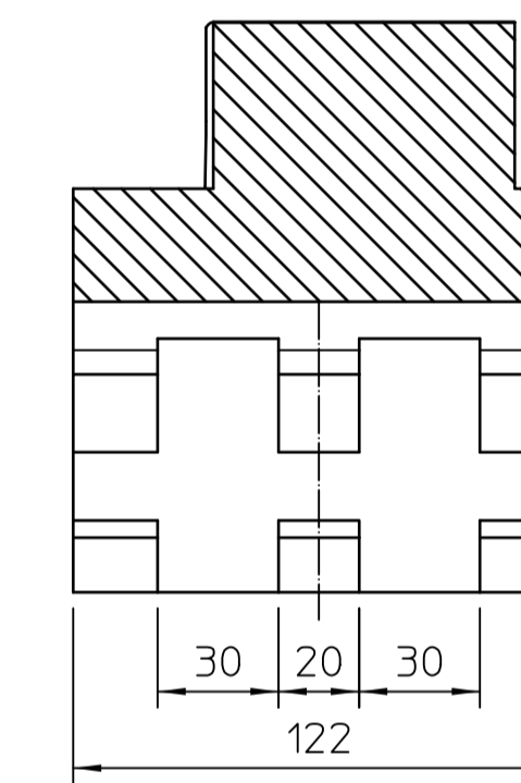
Schnitt B-B
