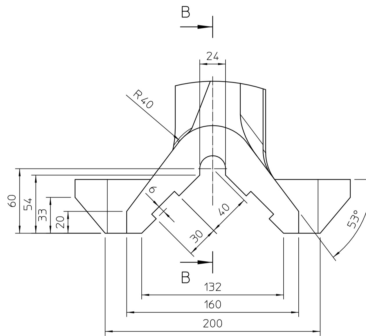
Teilansicht2 Maßstab 1:2
