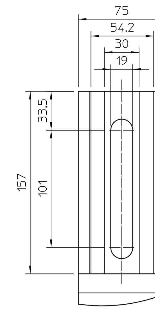
Teilansicht1 Maßstab 1:2
